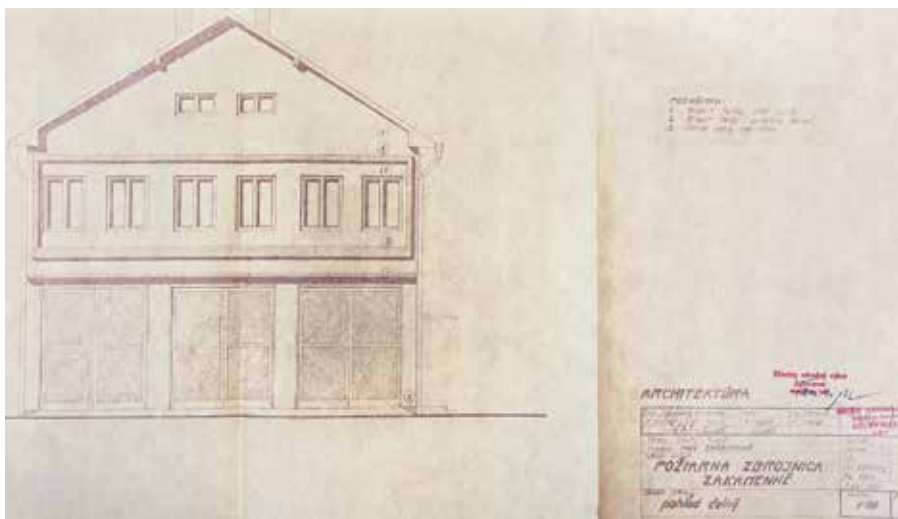
Plán požiarnej zbrojnice z roku 1972 (Archív Dolný Kubín)
